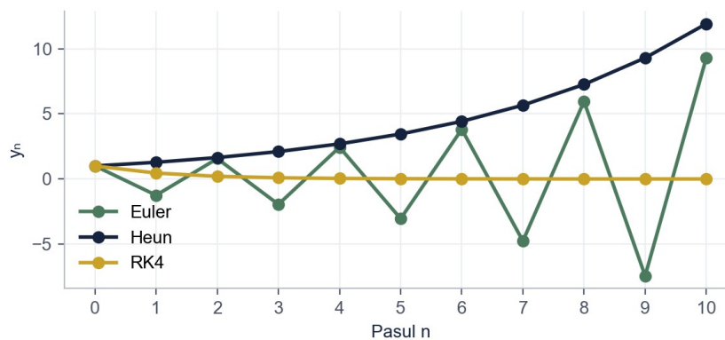
Figura 7. Aproximațiile pentru y' = -15y cu pasul h = 0,15 (primii 10 pași)
