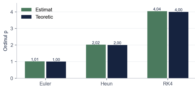
Figura 5. Ordinul de convergență estimat (perechea 0,025 → 0,0125) și ordinul teoretic Sursa: Prelucrare proprie după Tabelul 6.
