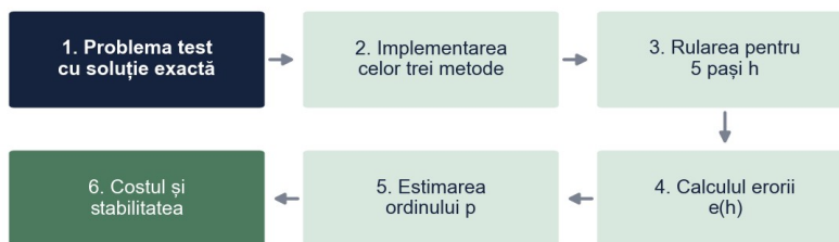
Figura 2. Etapele experimentului numeric
