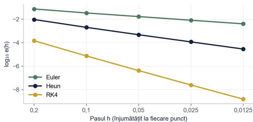
Figura 4. Logaritmul zecimal al erorii globale maxime, în funcție de pas
