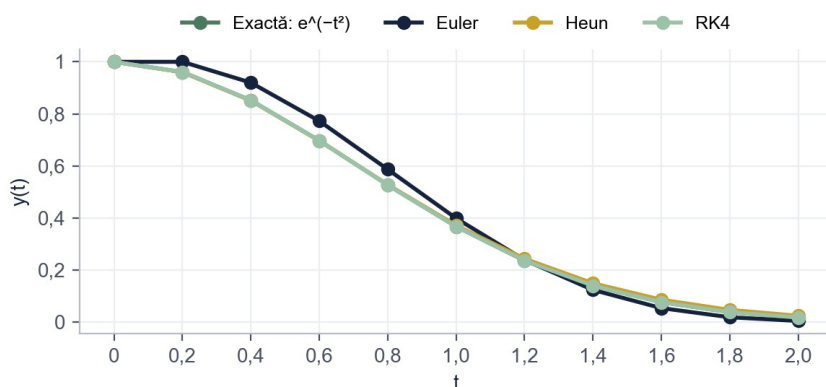
Figura 3. Soluția exactă și aproximațiile obținute cu pasul h = 0,2
