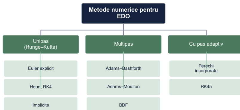
Figura 1. Clasificarea metodelor numerice pentru problema Cauchy
