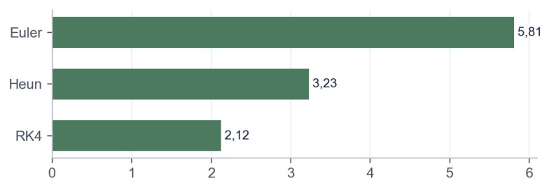
Figura 6. Numărul de evaluări ale lui f pentru e(h) < 10^{-6} (logaritm zecimal)
