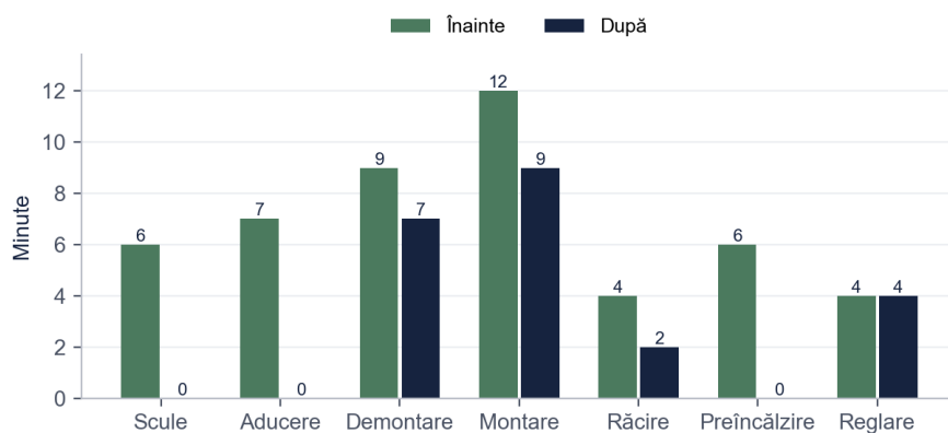
Figura 6. Durata operațiilor interne ale schimbării de matriță, înainte și după SMED (min)
