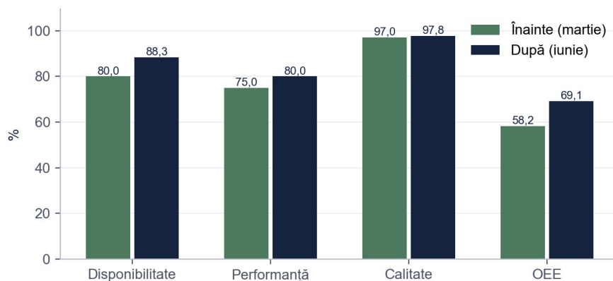
Figura 7. Componentele OEE înainte și după implementarea măsurilor (%)
