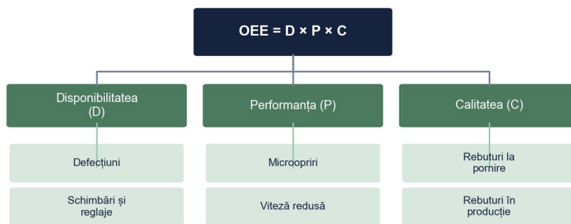
Figura 1. Structura indicatorului OEE și pierderile corespunzătoare
