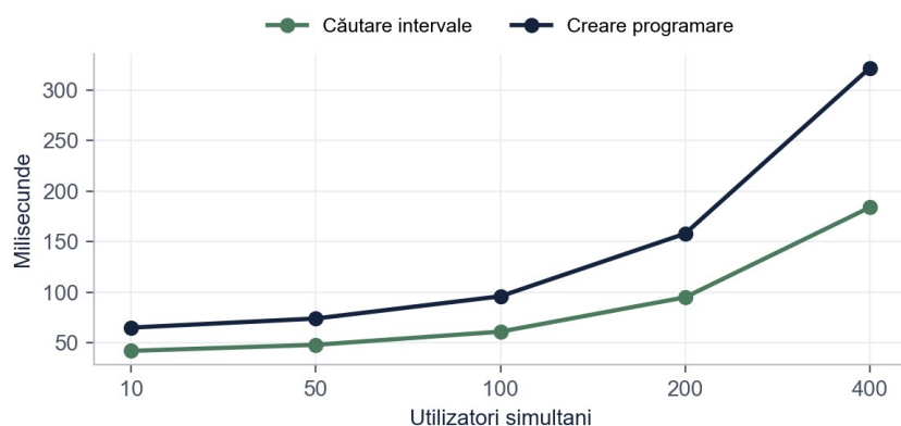
Figura 6. Timpul mediu de răspuns sub încărcare
