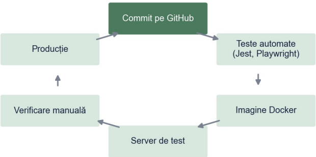
Figura 4. Fluxul de integrare și livrare continuă (CI/CD) folosit în proiect
