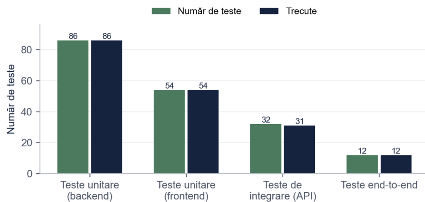
Figura 5. Testele automate, pe tipuri
