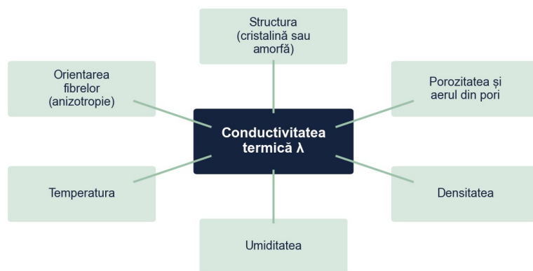
Figura 1. Factorii care influențează conductivitatea termică a unui material
