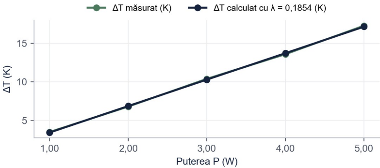
Figura 5. Diferența de temperatură în funcție de puterea aplicată (PMMA)
