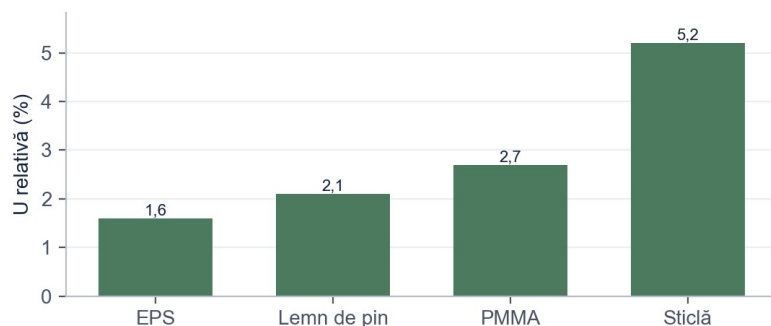
Figura 7. Incertitudinea extinsă relativă ( k = 2 ), pe materiale (%)
