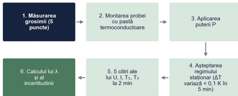
Figura 3. Etapele unei măsurători
