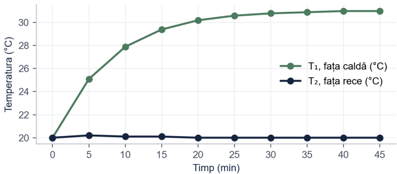
Figura 4. Atingerea regimului staționar pentru proba de PMMA ( P \approx 3,2 \text{ W} ) Sursa: Măsurători de laborator (valori simulate pentru exemplu).
