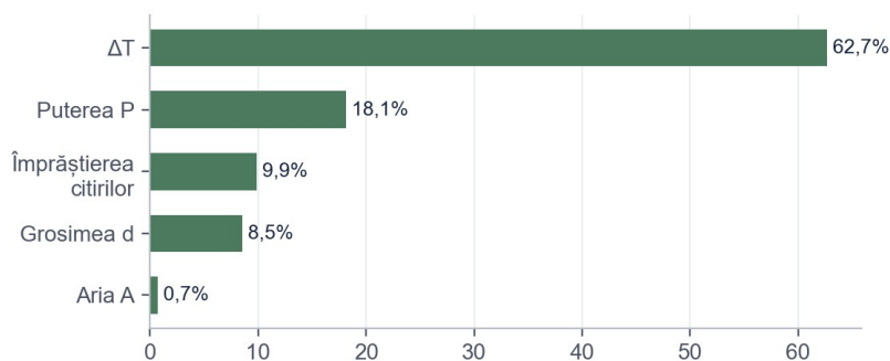
Figura 6. Contribuțiile la varianța lui \lambda pentru proba de PMMA (%)
