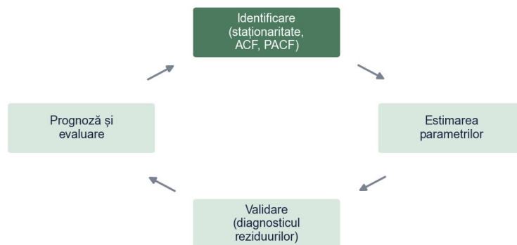
Figura 1. Etapele metodologiei Box–Jenkins
