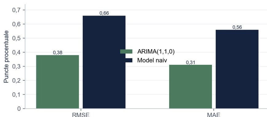
Figura 8. Erorile de prognoză: ARIMA(1,1,0) și modelul naiv (puncte procentuale)
