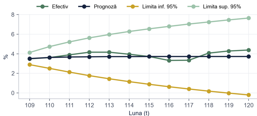
Figura 7. Prognoza ARIMA(1,1,0) și valorile efective în lunile 109–120 (%)
