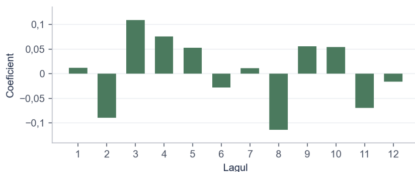
Figura 6. Autocorelațiile reziduurilor modelului ARIMA(1,1,0), lagurile 1–12 (pragul \pm 0,19 )
