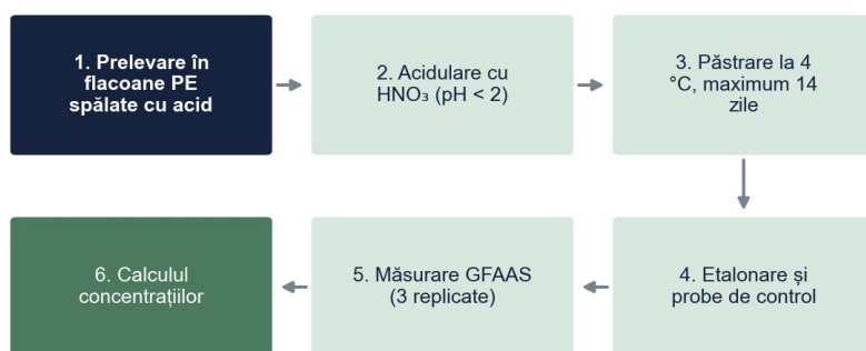
Figura 3. Etapele procedurii experimentale
